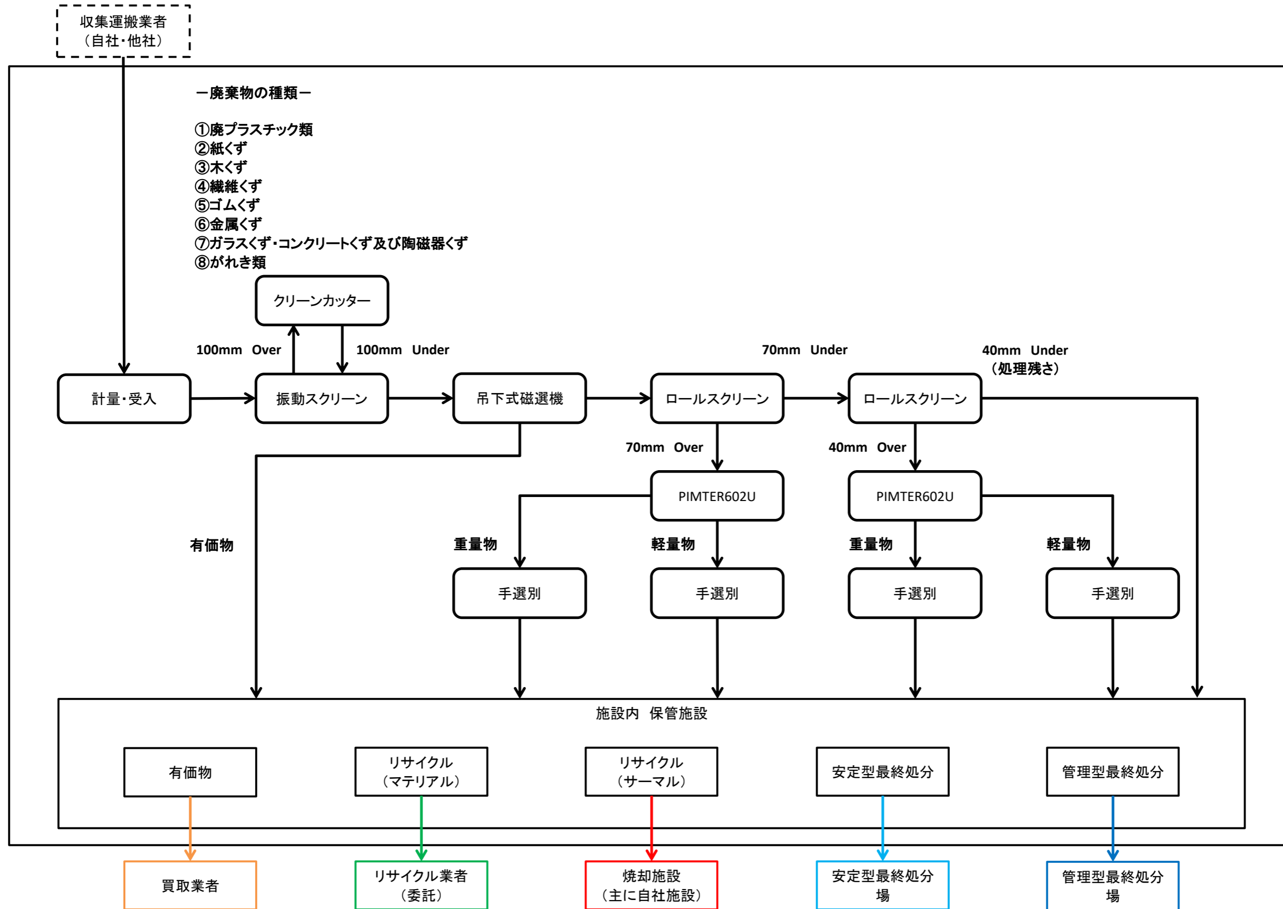
○事業場ごとの産業廃棄物の処理工程図(坂下事業所)
